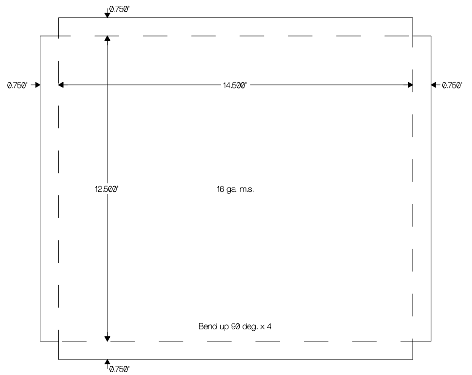
Lid Layout
